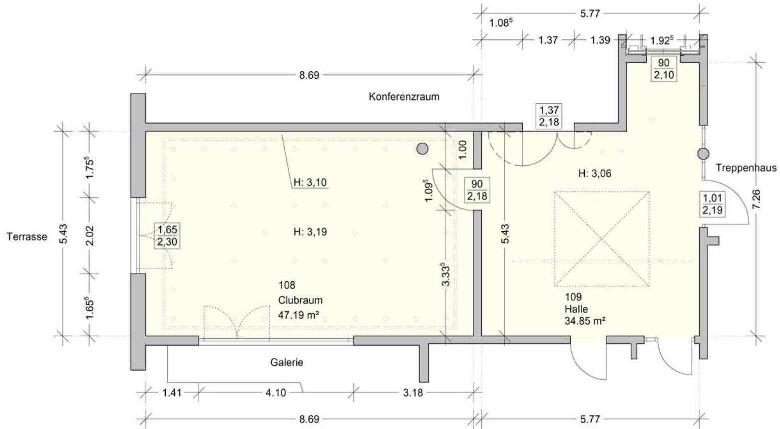
HÖHENSHEMA DECKE 108
