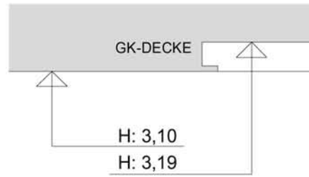
HÖHENSHEMA DECKE 108
